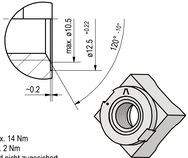
Einzelheit X ( 4 : 1 )
